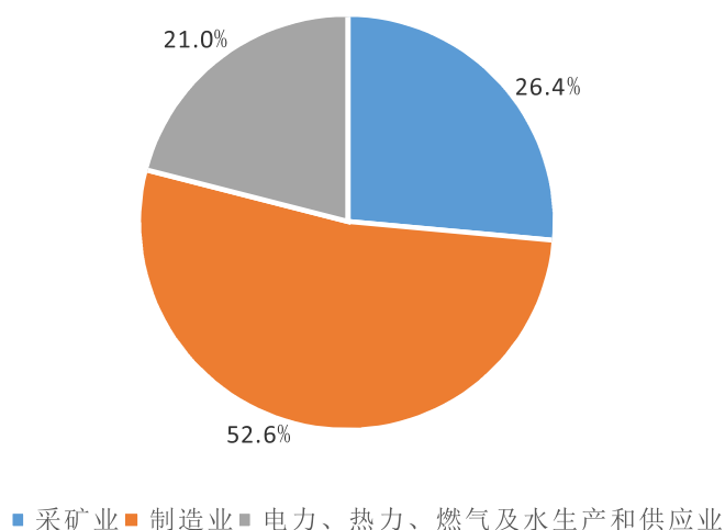
2025年铁岭市规模以上工业增加值行业构成
