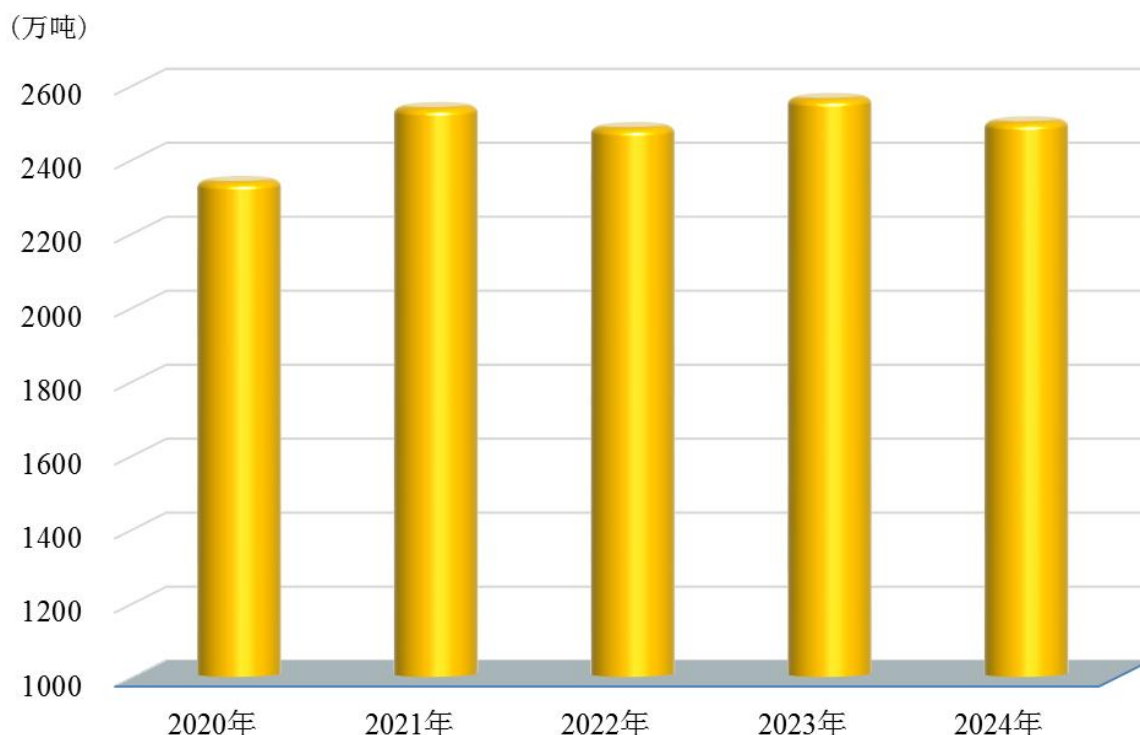
图 1 2020-2024 年粮食产量
