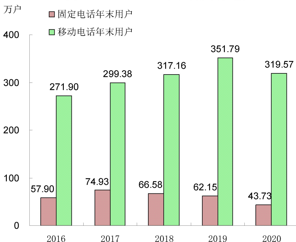
图12 2016-2020年末电话用户数
