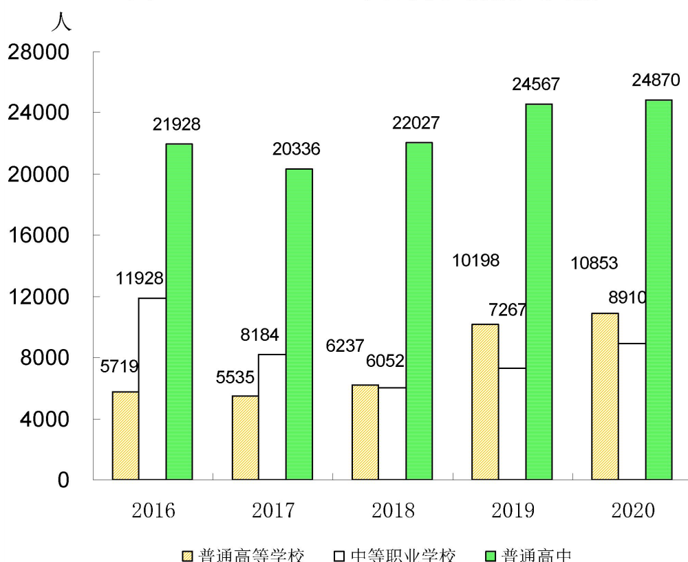
图14 2016-2020年各类学校招生人数
