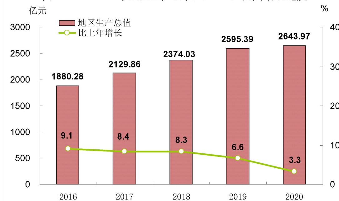
图1 2016-2020年地区生产总值（GDP）及其增长速度
